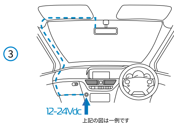
ケーブル設置ツール(パッケージに付属)
